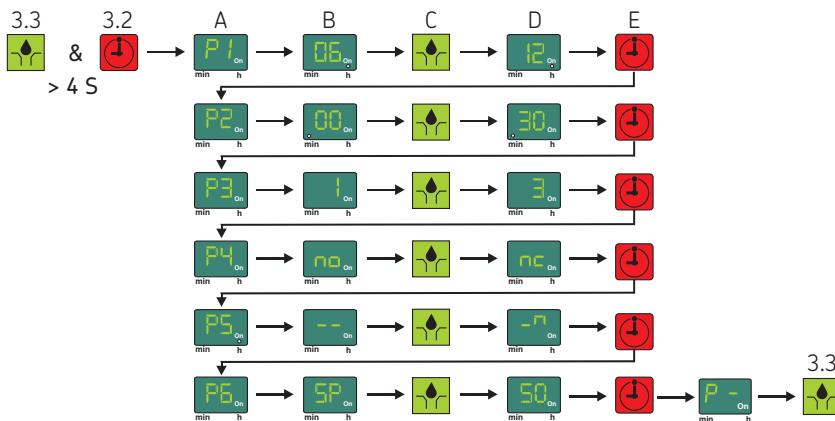
编程方案图，图 10
