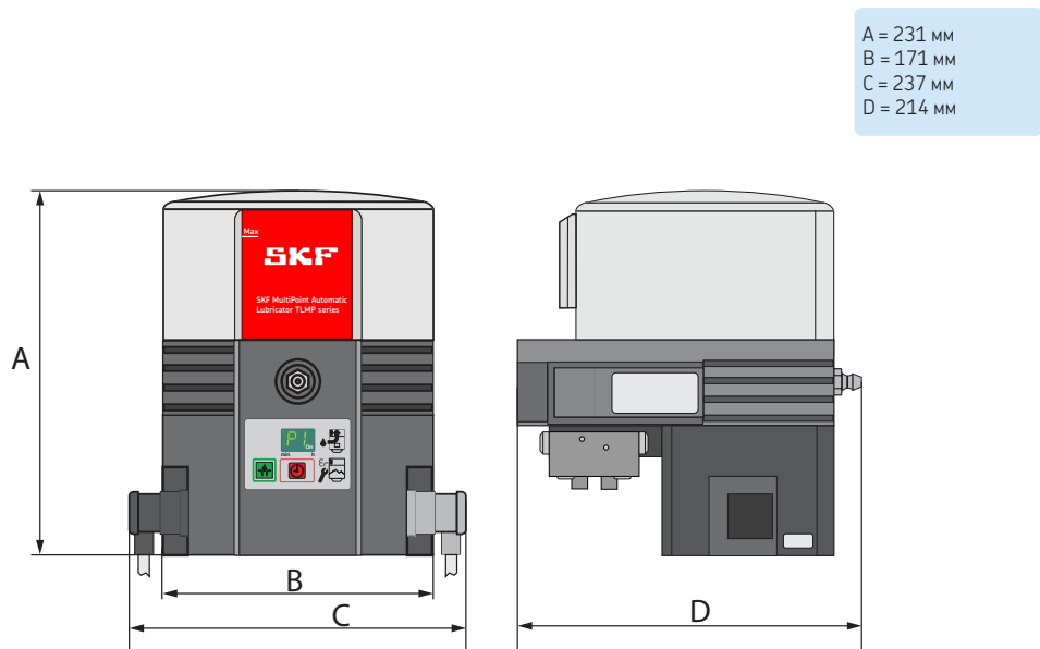
Рис. 6. Минимальные установочные размеры
